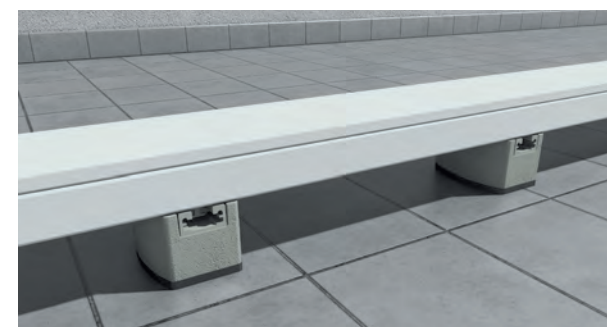
Perfil Ω perforado metálico disponible en: · Acero inox. AISI 304 con pintura epoxy gris. · Acero galvanizado con pintura epoxy gris. Con soportes horizontales aislantes en U48X.
