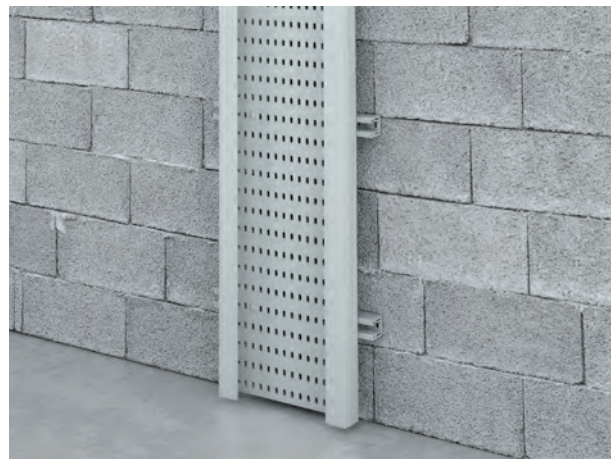
Soporte L disponible en: · Acero sendzimir. · Acero galvanizado con pintura epoxy gris.
